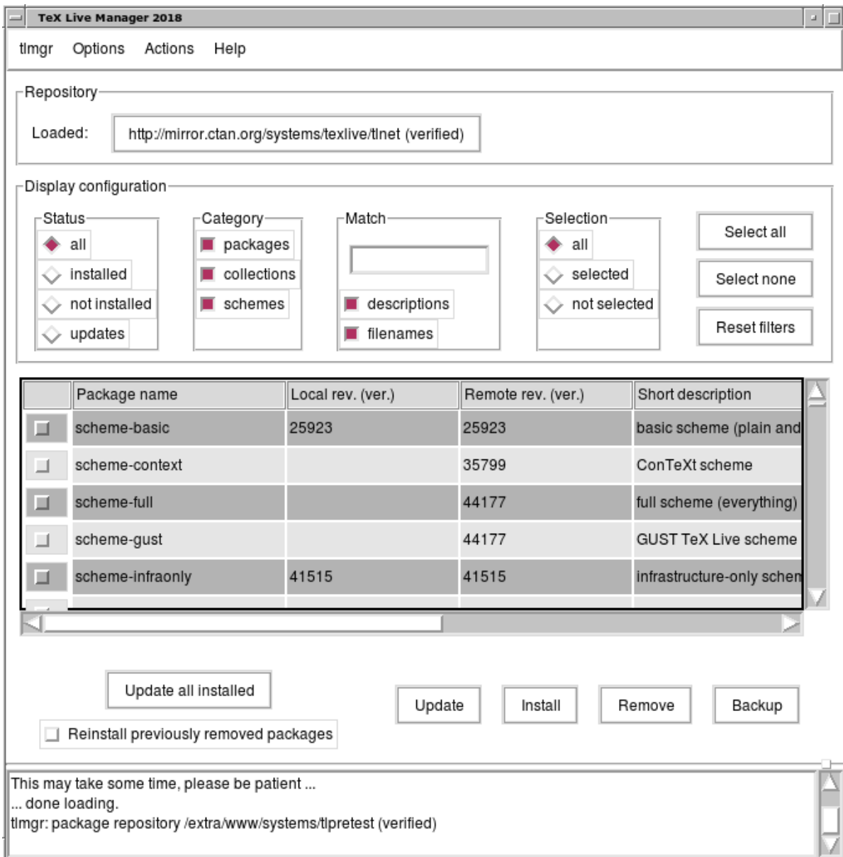
Figura 11: Modalità GUI obsoleta di tlmgr: finestra principale dopo aver premuto il pulsante ‘Carica’
