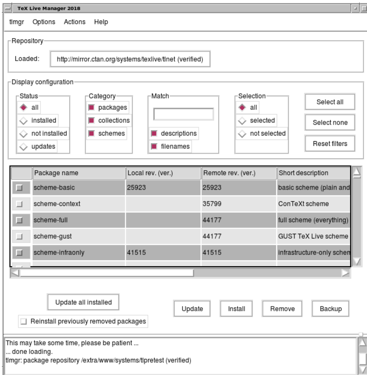
Obrázek 11: Starší režim tlmgr GUI: hlavní okno, po kliknutí na tlačítko ‚Load‘
