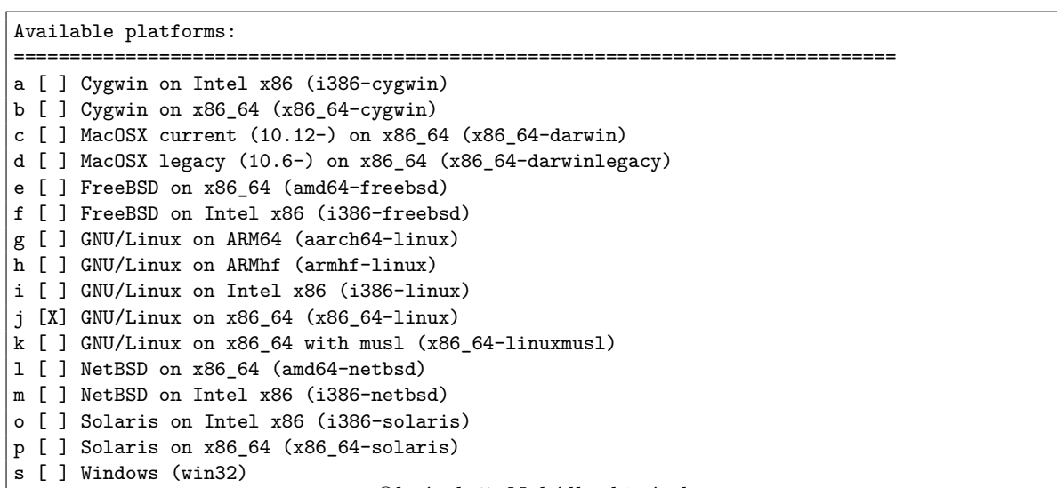
Obrázek 5: Nabídka binárek
