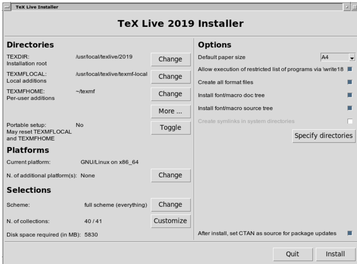
Obrázek 4: Obrazovka pokročilého GUI instalátoru (GNU/Linux)
